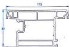
Casement Door Sash-115
